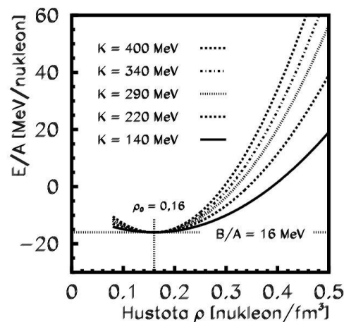
Obr.1. Stavová rovnice jaderné hmoty E/A = f(\rho) při teplotě T = 0 K pro různé varianty tvrdosti (parametru stlačitelnosti). 3
