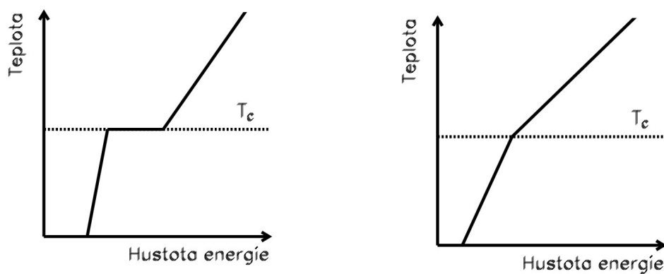
Obr. 4. a) Fázový přechod prvního druhu b) Fázový přechod druhého druhu
