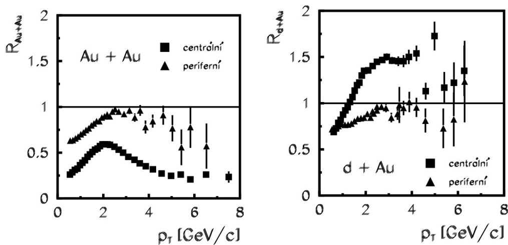
Obr. 11. Rozdíl v produkci výtrysků (nabitých částic) s velkou příčnou hybností p_T mezi srážkami zlata se zlatem a deuteronu se zlatem (normováno na produkci v jedné srážce nukleonu s nukleonem vynásobenou počtem takových srážek). Data byla získána díky experimentu PHOENIX pro centrální a periferní srážky. U srážek Au + Au se u centrálních srážek projevuje jak potlačení pohybem v kvark-gluonové plazmě, tak i Croninův jev. U srážek d + Au se projevuje pouze vliv Croninova jevu.
