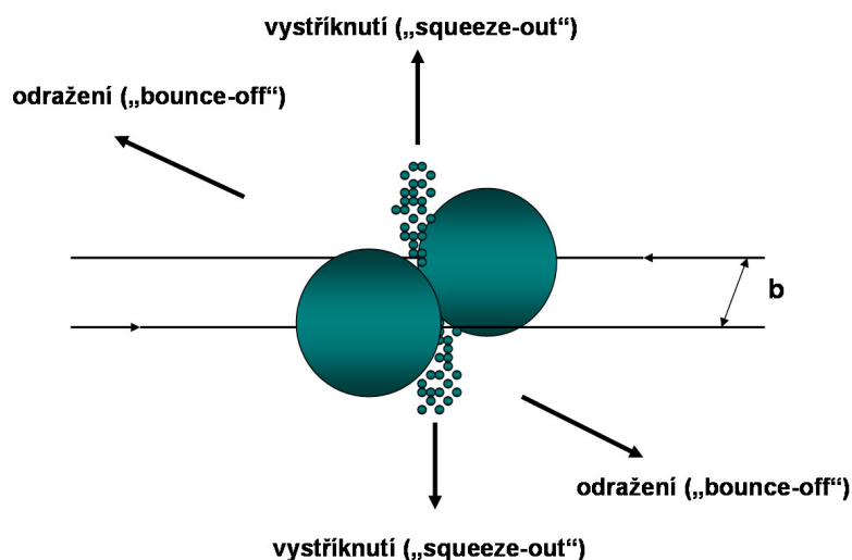
Obr. 6. Kolektivní toky částic.
