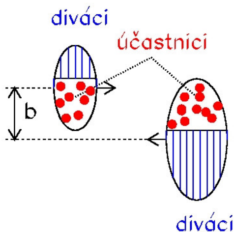
Obr. 5. Rozdělení nukleonů během srážky.
