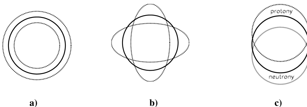
Obr. 2. Různé druhy změn tvaru jádra: a) změny objemu jádra, b) změny tvaru jádra, c) gigantické rezonance.
